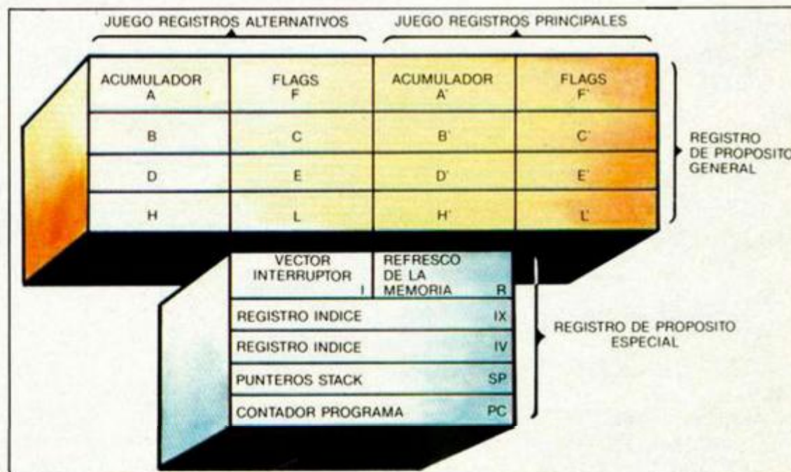
Figura 1: Registros de programación del Z-80.
